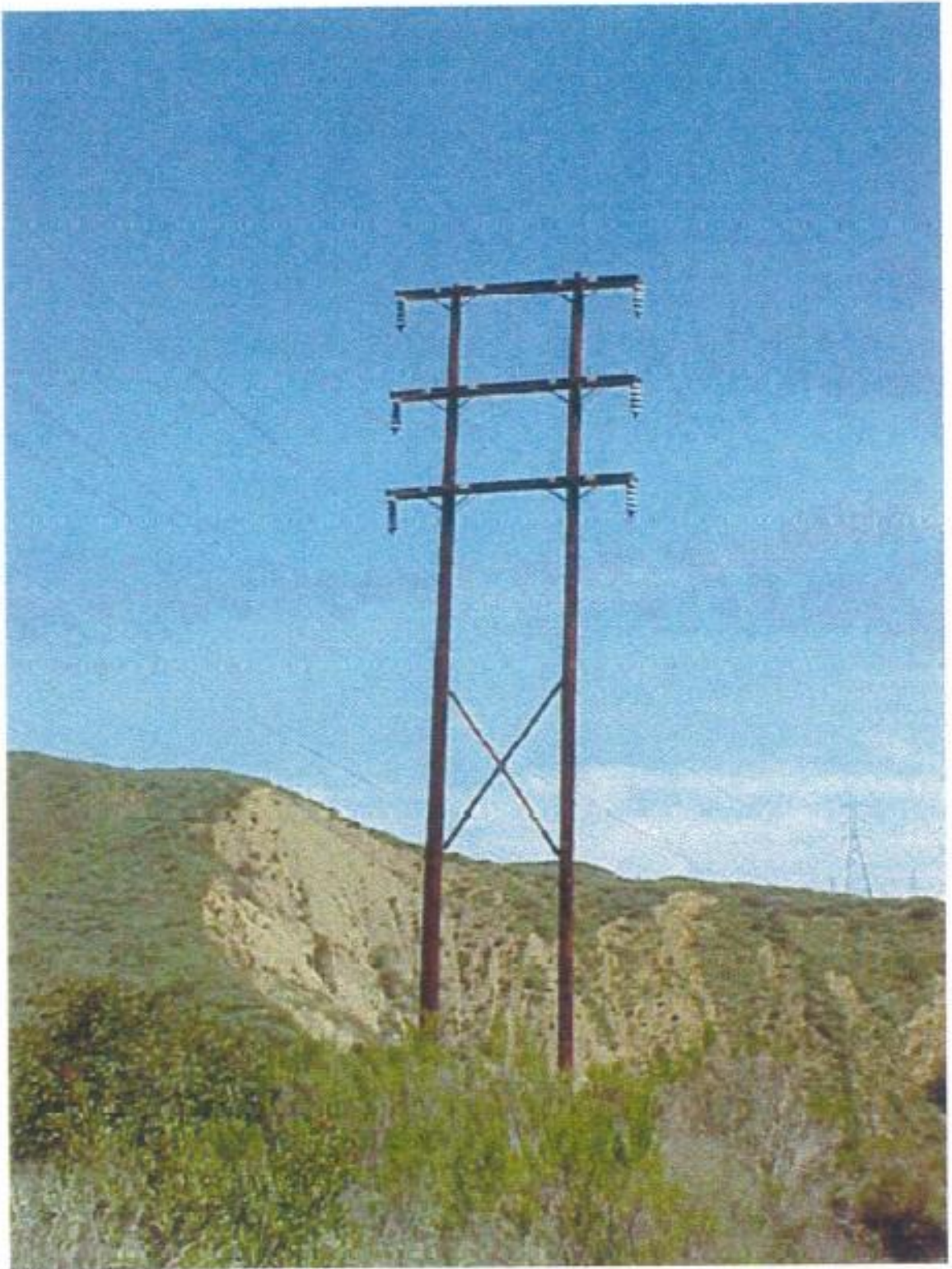
100' Wood H-Frame 1872175E &187216E
