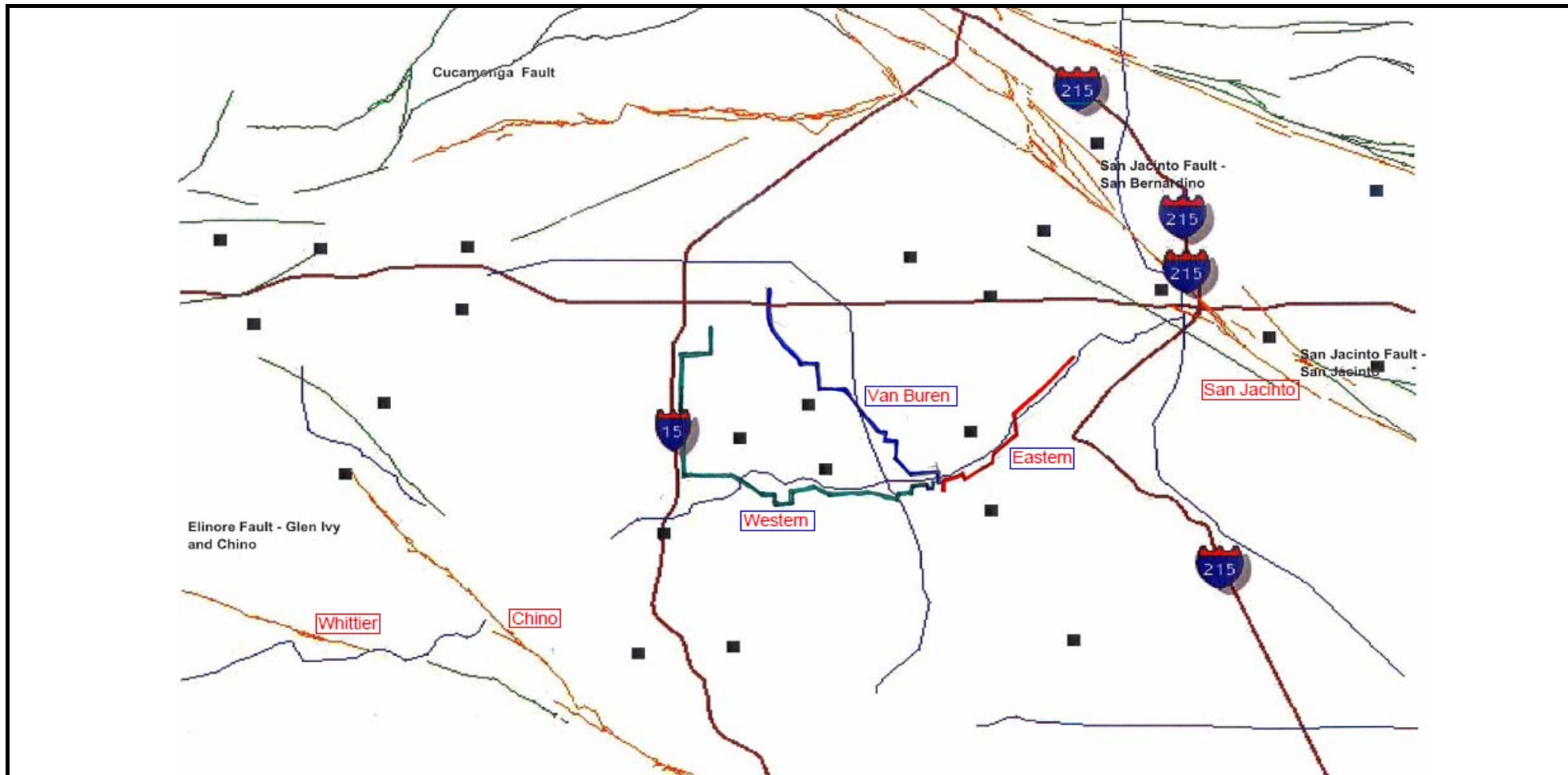
Faulting & Local Seismicity Map
